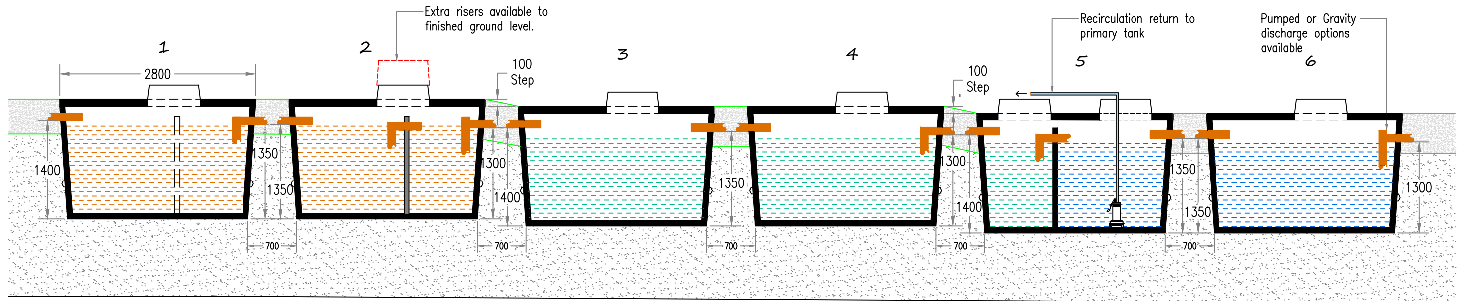
SECTION A-A
